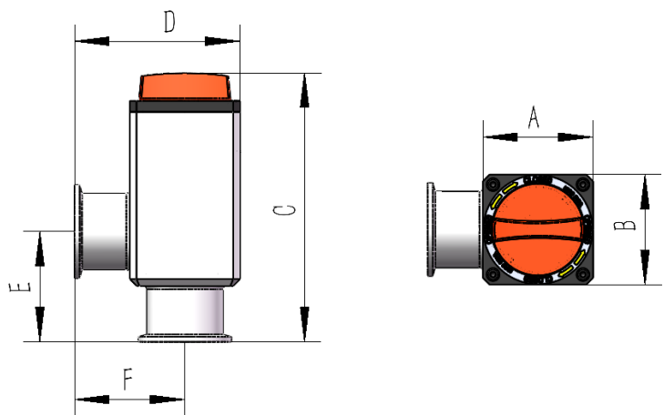
角阀尺寸表 (mm)
