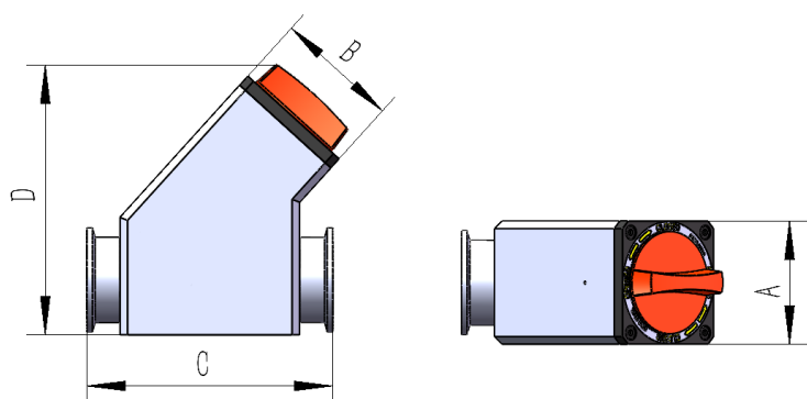
直通阀尺寸表 (mm)
